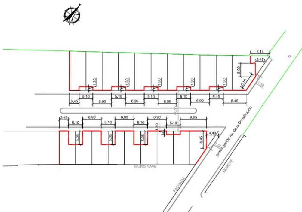
Plano alineaciones
